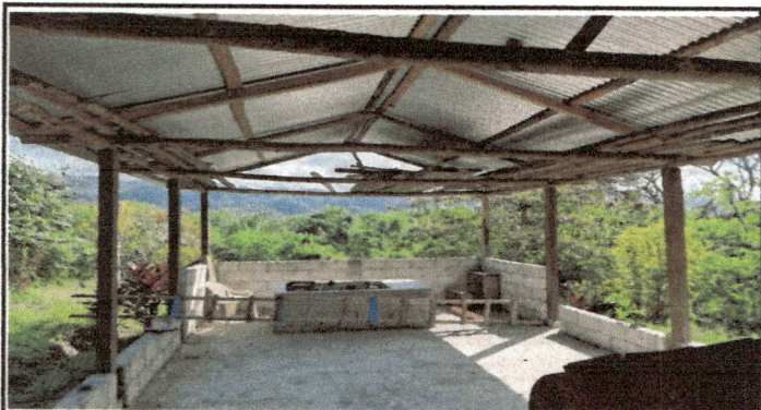
Foto 3: ESTRUCTURA DE TECHO. SUSTITUCIÓN DE ESTRUCTURA DE SOPORTE DE MADERA, POR METAL
